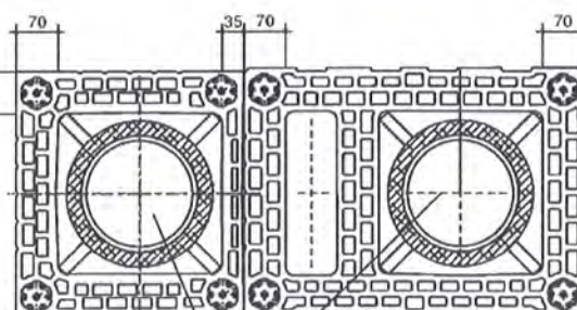
ZMS 42+ ZMS 42L ERLUS Ek - Rohr
