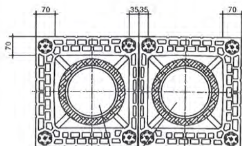
ZMS 42+ ZMS 42+ ERLUS Ek - Rohr
