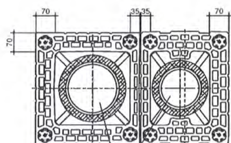
ZMS 42+ ZMS 42R+ ERLUS Ek - Rohr
