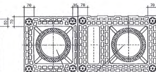
ZMS 42+ ZMS 42L ERLUS Ek - Rohr
