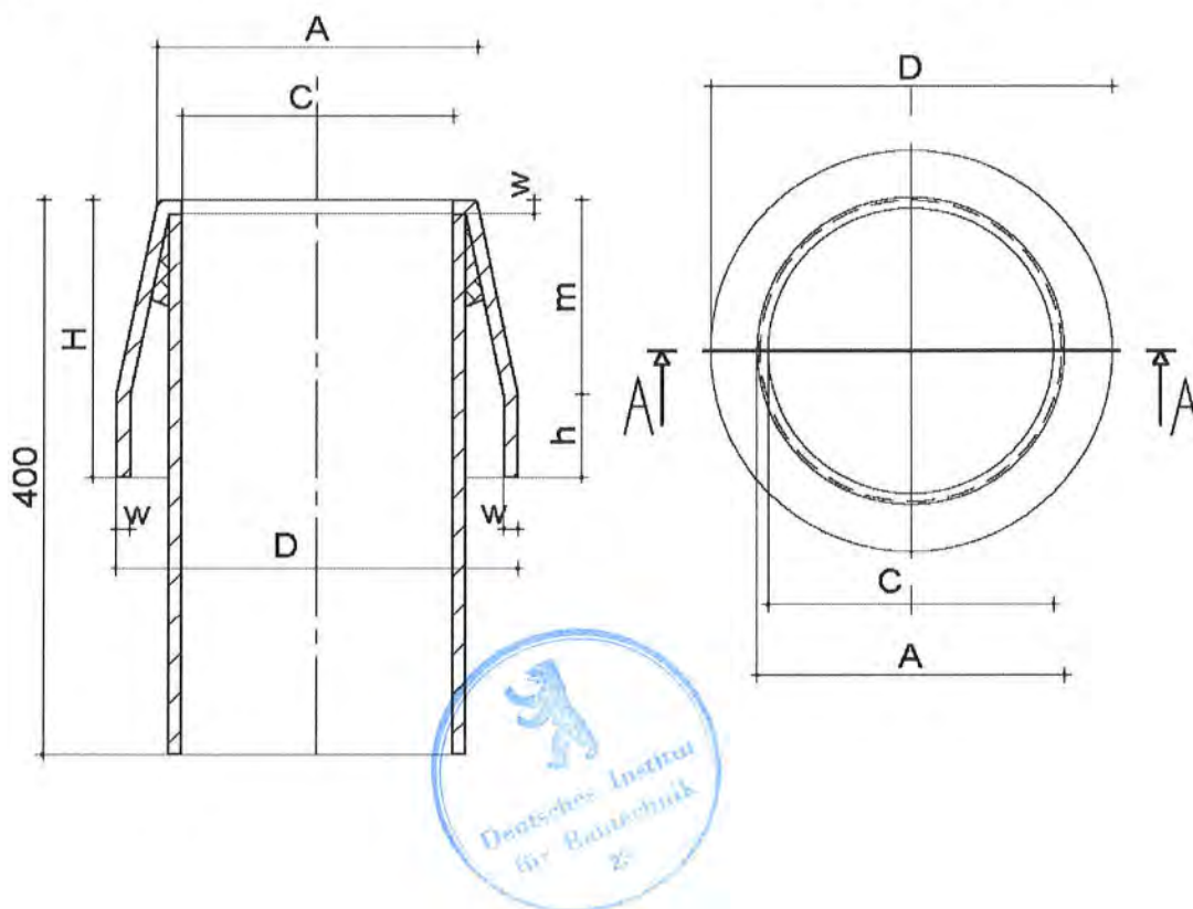
Maßtabelle in mm
