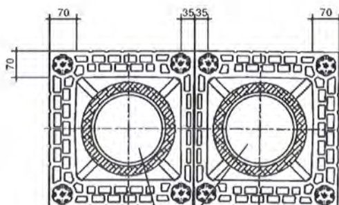
ZMS 42+ ZMS 42+ ERLUS Ek - Rohr
