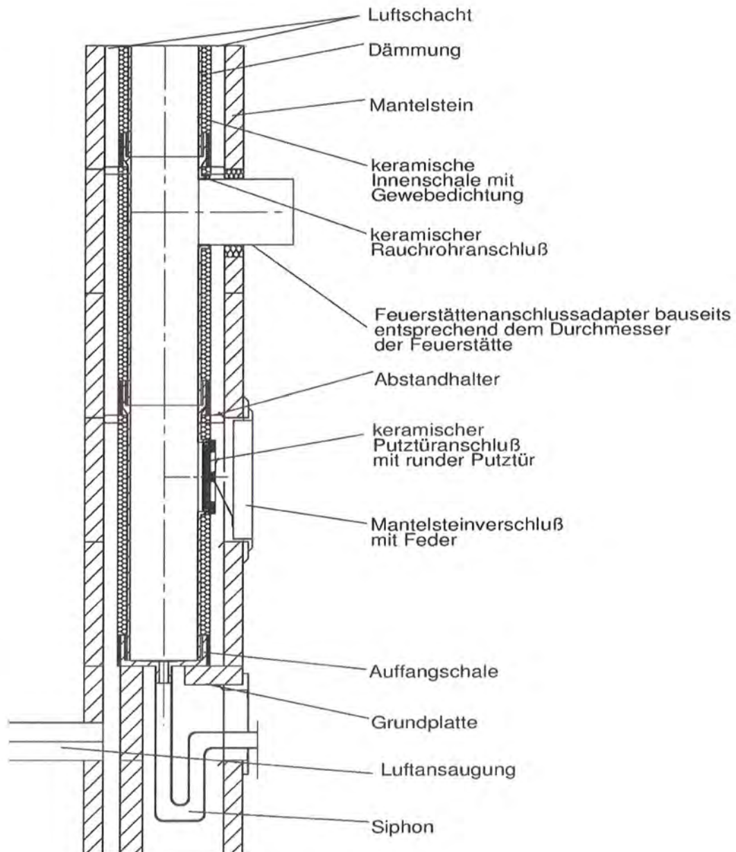
Variante der Fußausbildung zu Anhang 13
