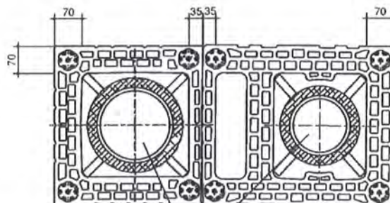
ZMS 42+ ZMS 42LR+ ERLUS Ek - Rohr
